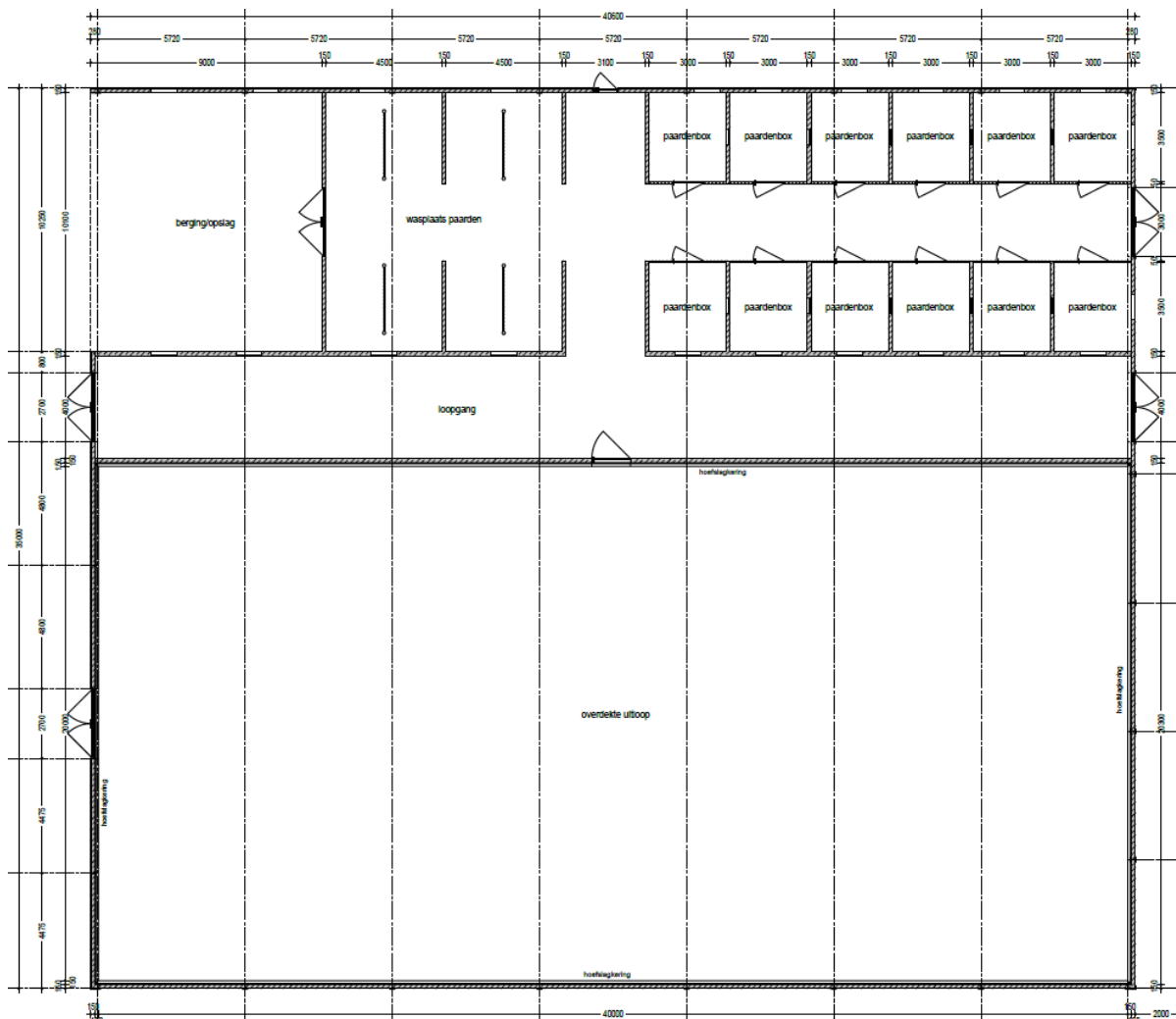
PLATTEGROND STALLEN/RIJBAK 35 X 40 METER
