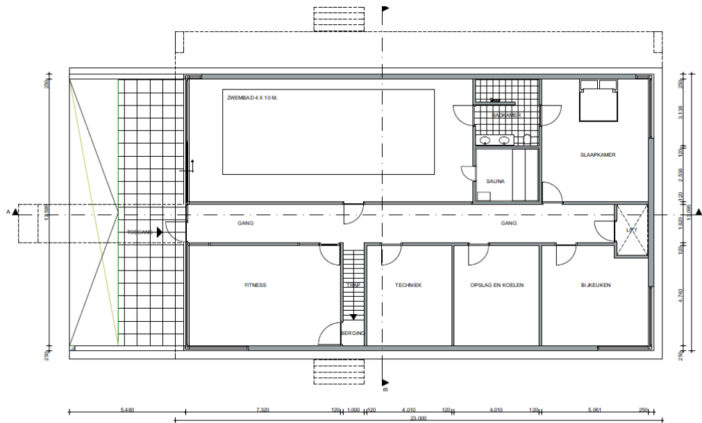
KELDER
