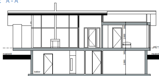
DOORSNEDE B-B
