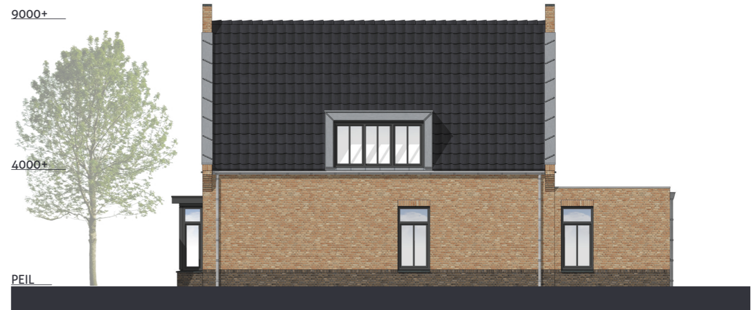
Zijgevel rechts
