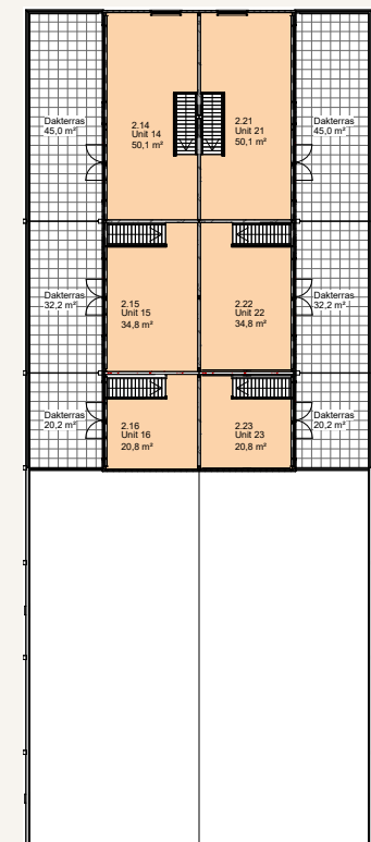
TWEEDE VERDIEPING
