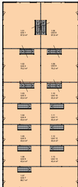
EERSTE VERDIEPING
