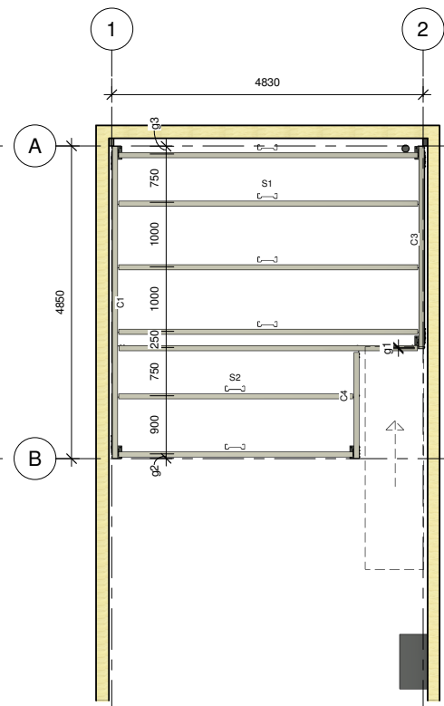
2 Staalconstructie 1 : 50
