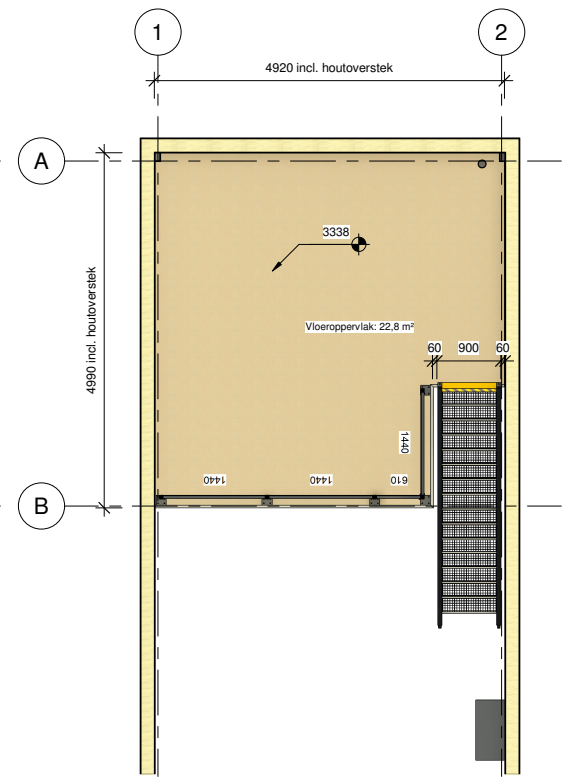
3 1e verdieping 1 : 50
