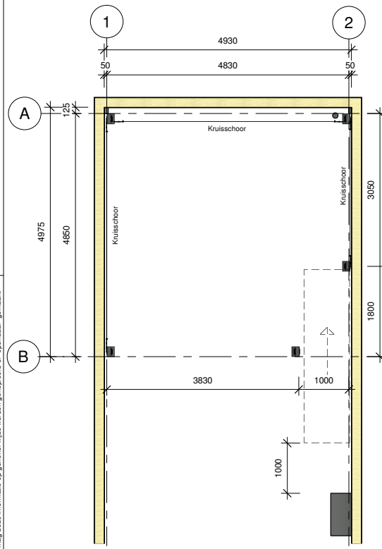
1 Begane grond 1 : 50
