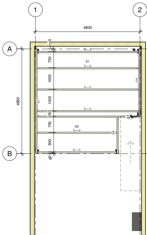
2 Staalconstructie
