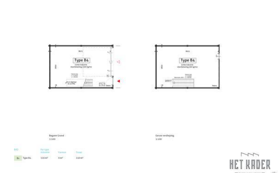
type B4 plattegronden
