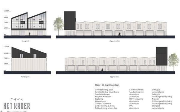
ontwerp aanzichten Blok B
