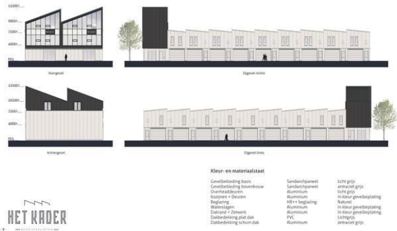
ontwerp aanzichten Blok B
