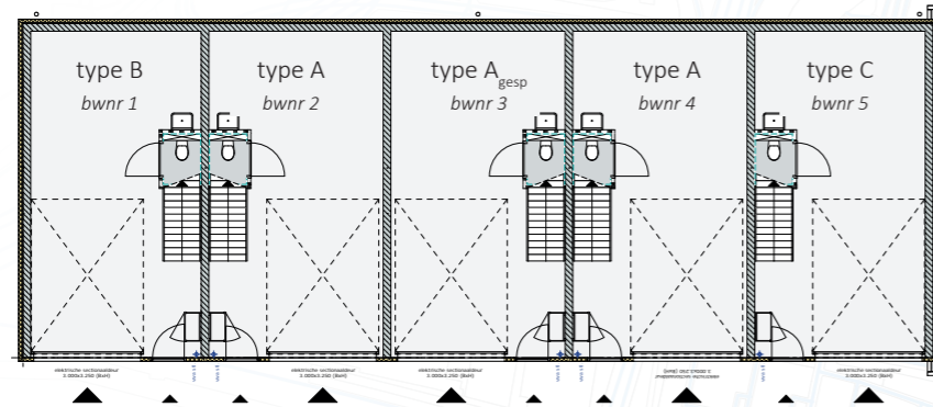
begane grond
