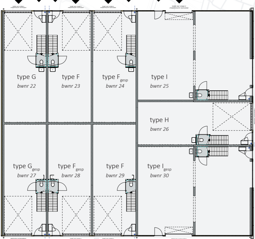
begane grond
