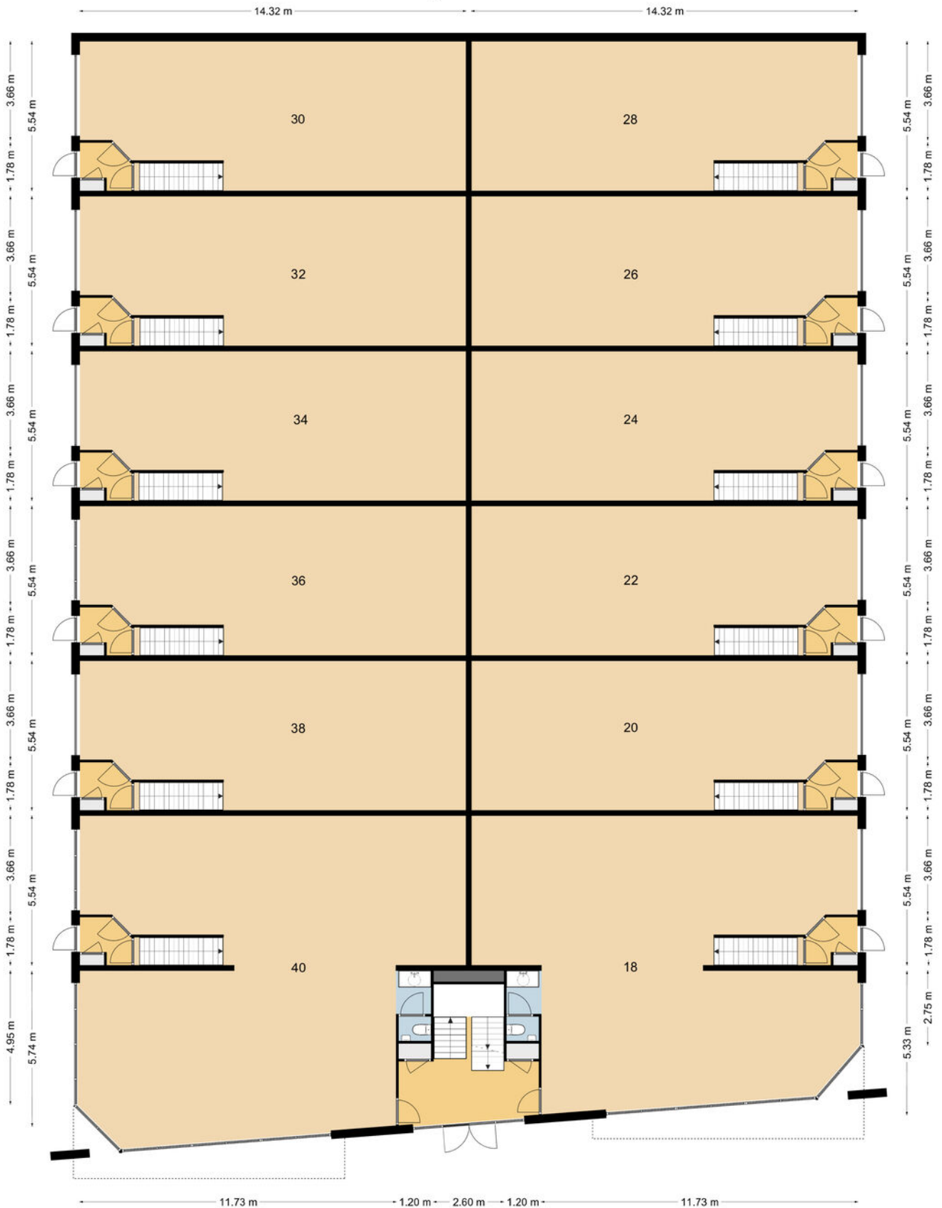
Begane Grond
