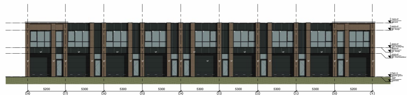
RECHTERZIJAANZICHT GEBOUW B
