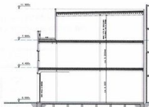
DWARSDOORSNEDE UNIT BOUWNUMMER 37t/m59
