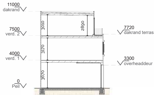
doorsnede 1
