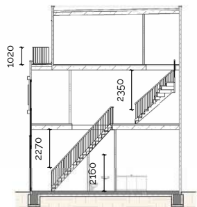
doorsnede 2
