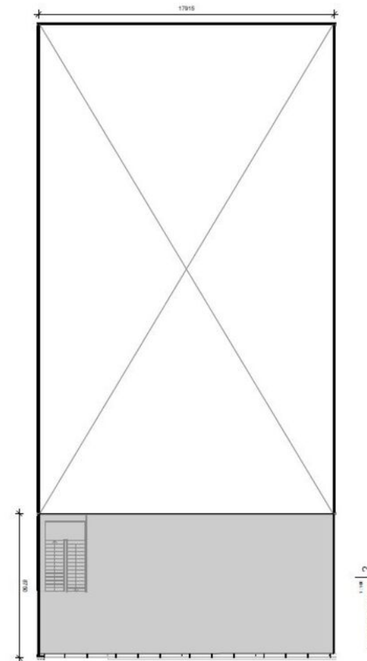
1e verdieping - Bouwdeel C BVO: 156 m 2
