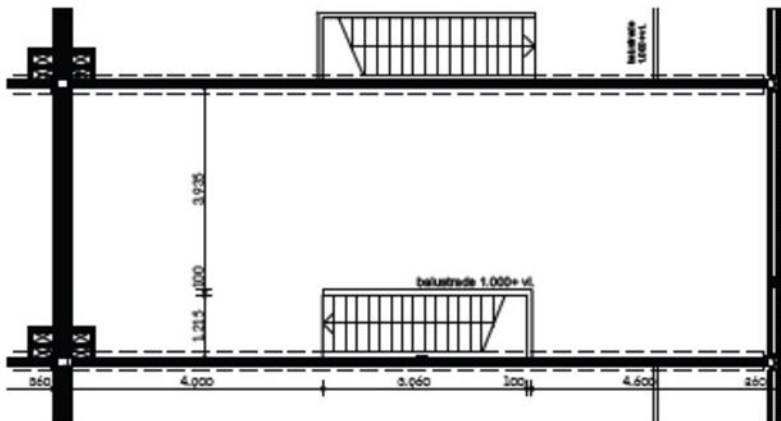
1e verdieping - variant met gedraaide trap
