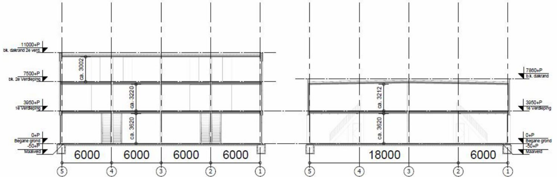
Doorsnede A
