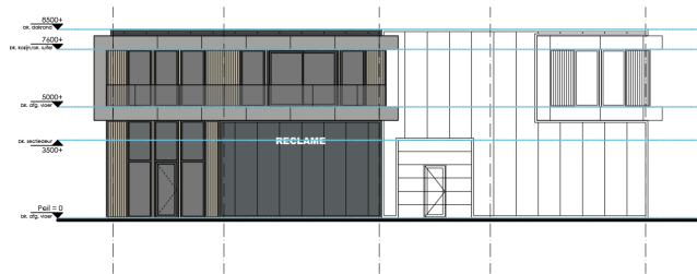
Noordgevel Pand A
