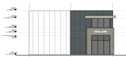
Noordgevel Pand C
