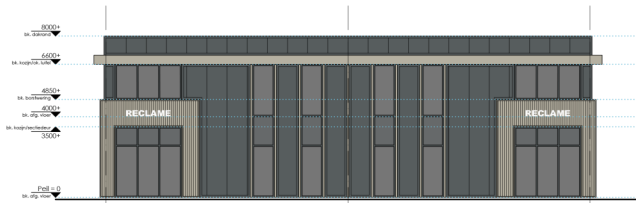
Noordgevel Pand B
