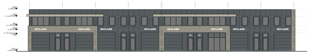
Westgevel Pand B
