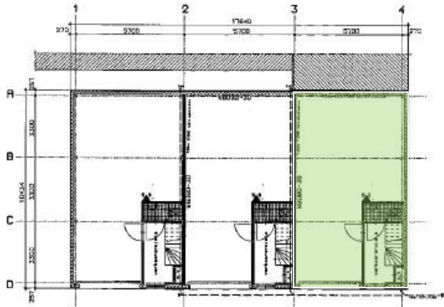
plaattegrond nivo 0.00
