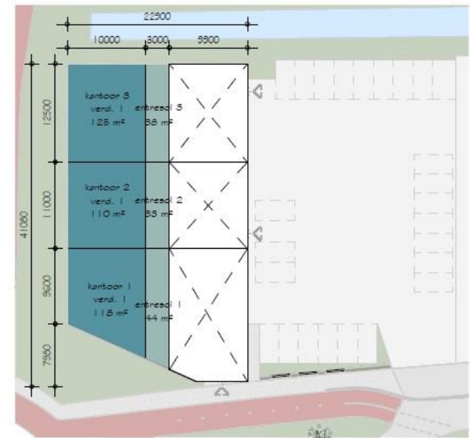
eerste verdieping (3950+)
