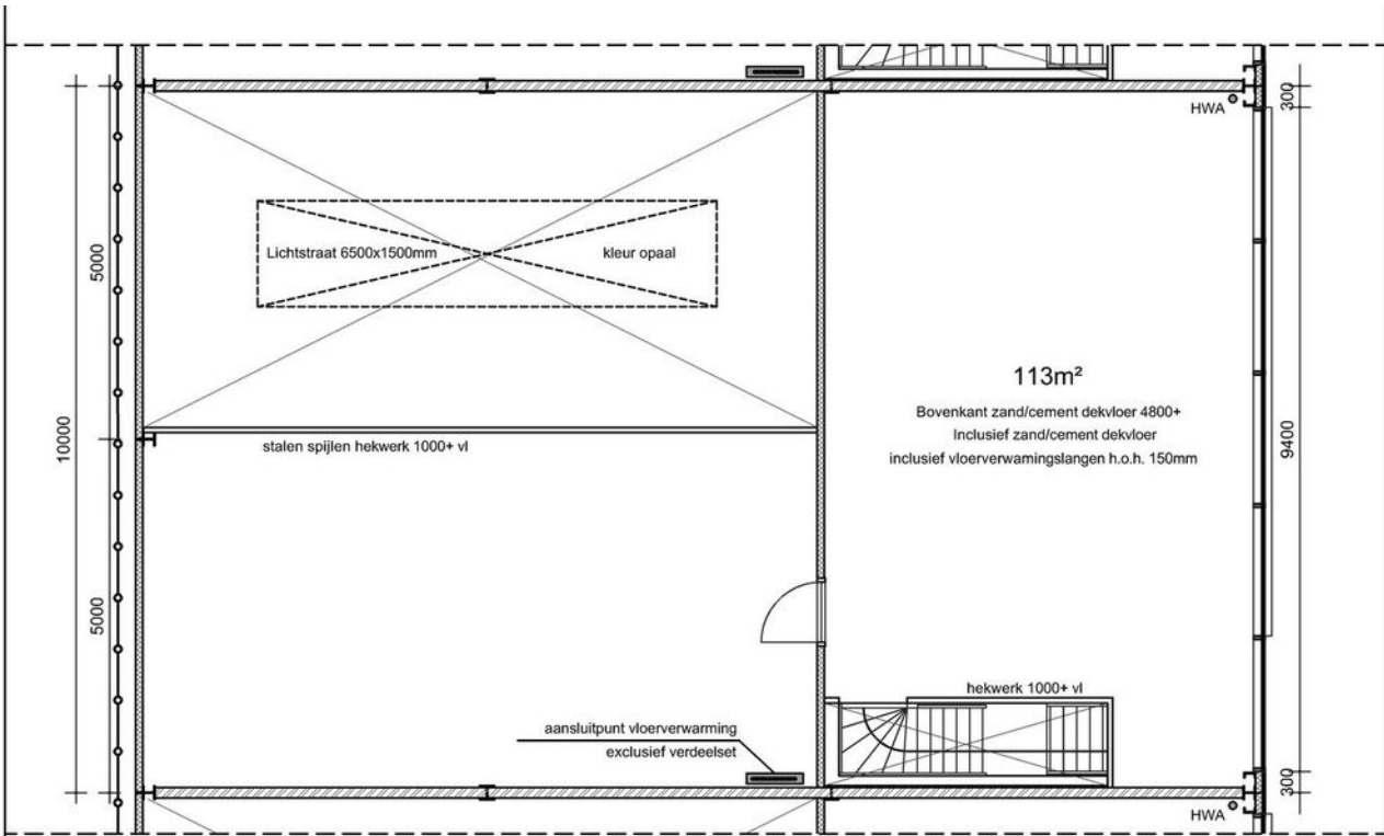
Eerste verdieping
