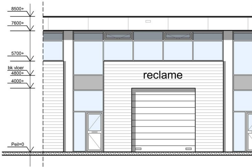
Voorgevel
