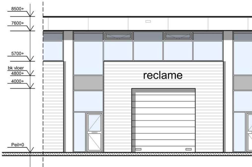
Voorgevel
