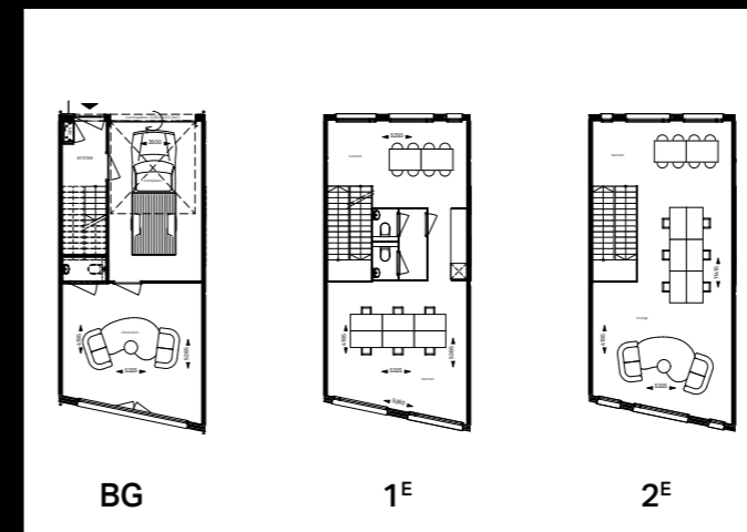
UNIT A - ENKELE UNIT
