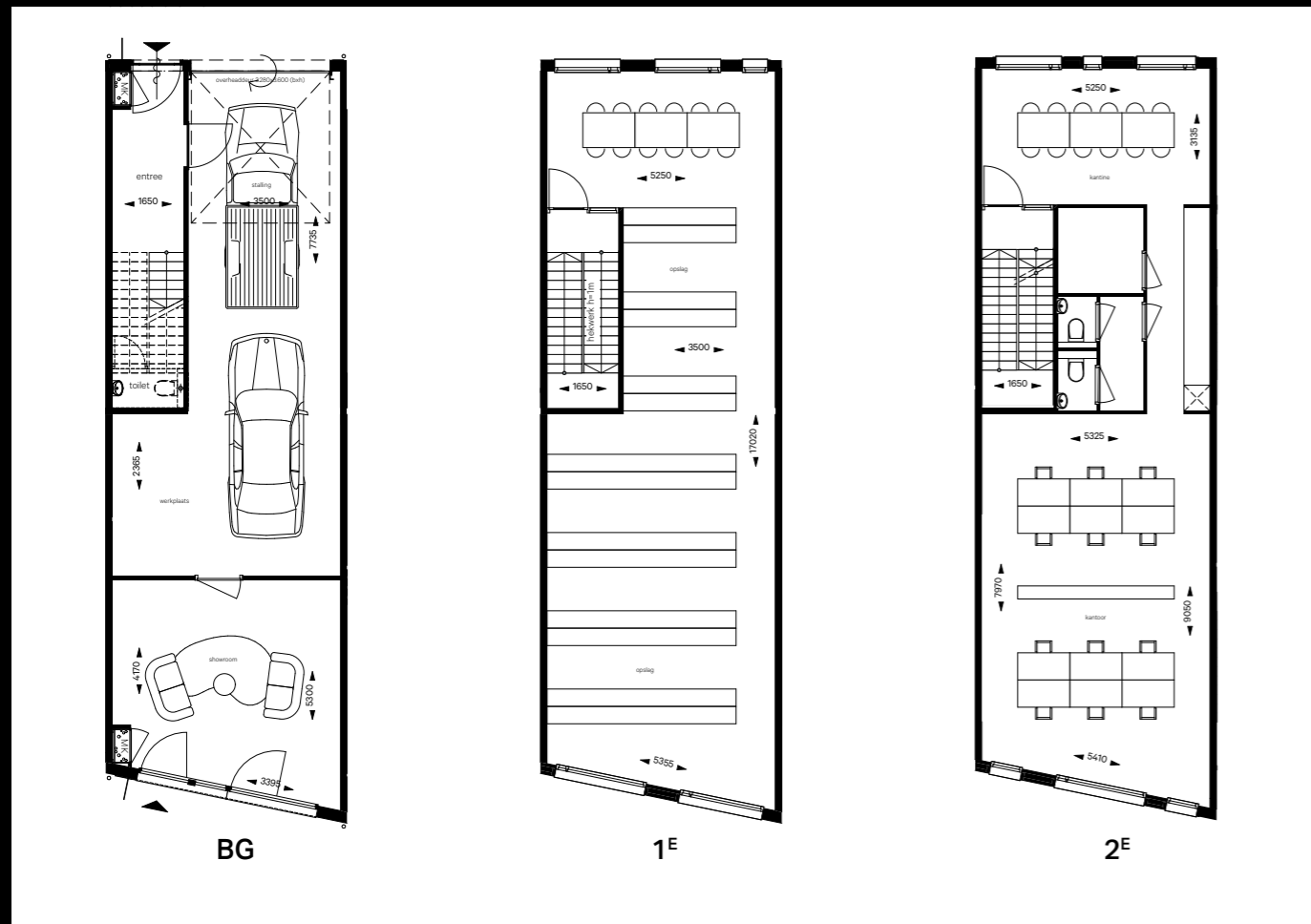
UNIT A - DUBBELE UNIT
