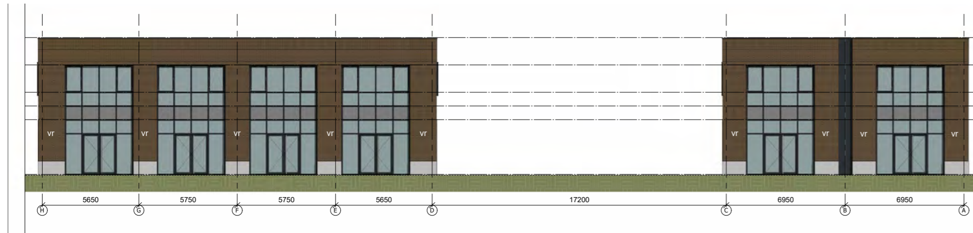
VOORGEVEL
