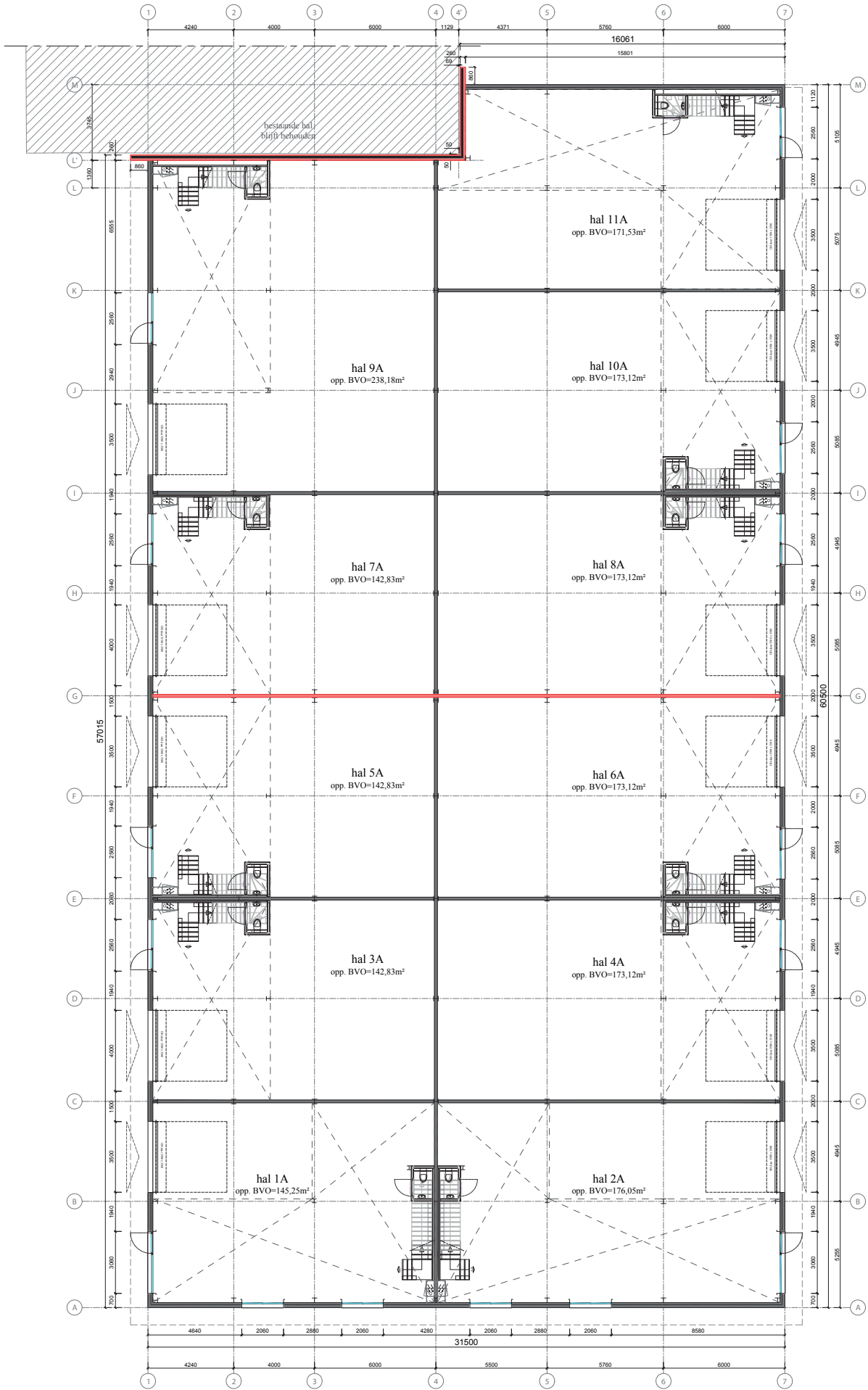
Grondplan
