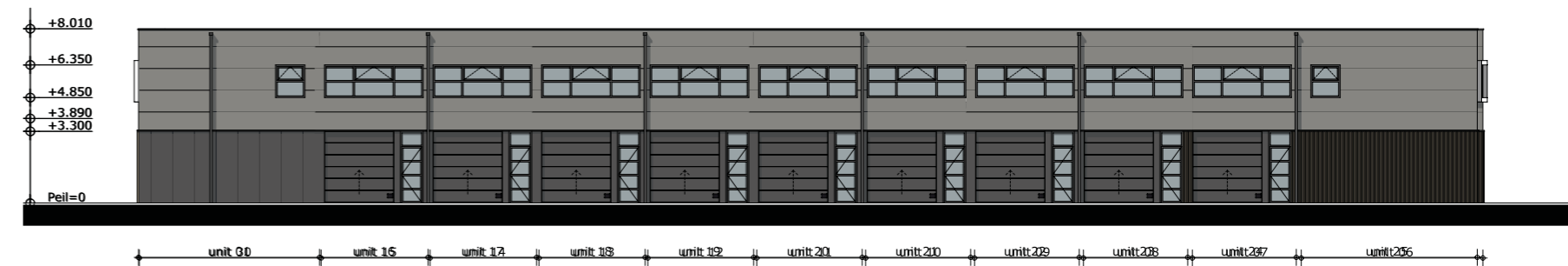
Zuidgevel
