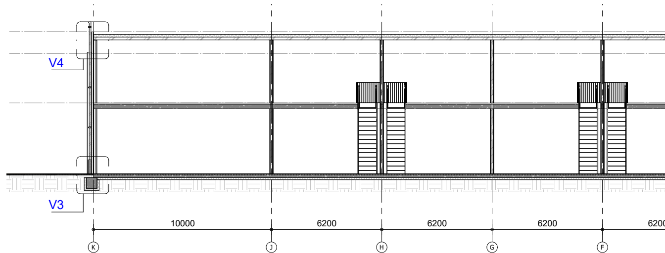
Doorsnede B-B
