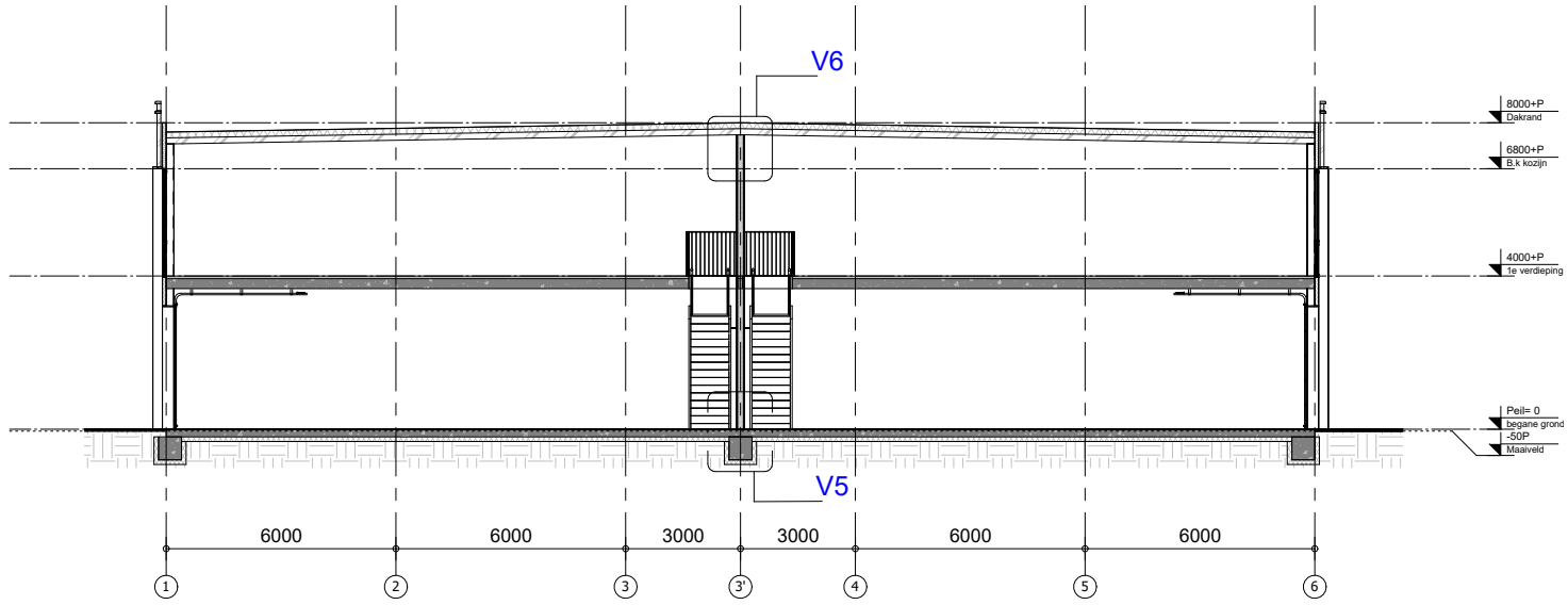
Doorsnede C-C
