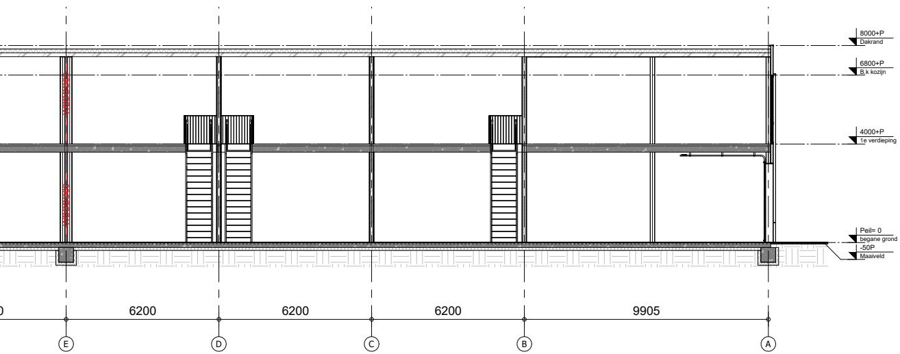
Doorsnede C-C
