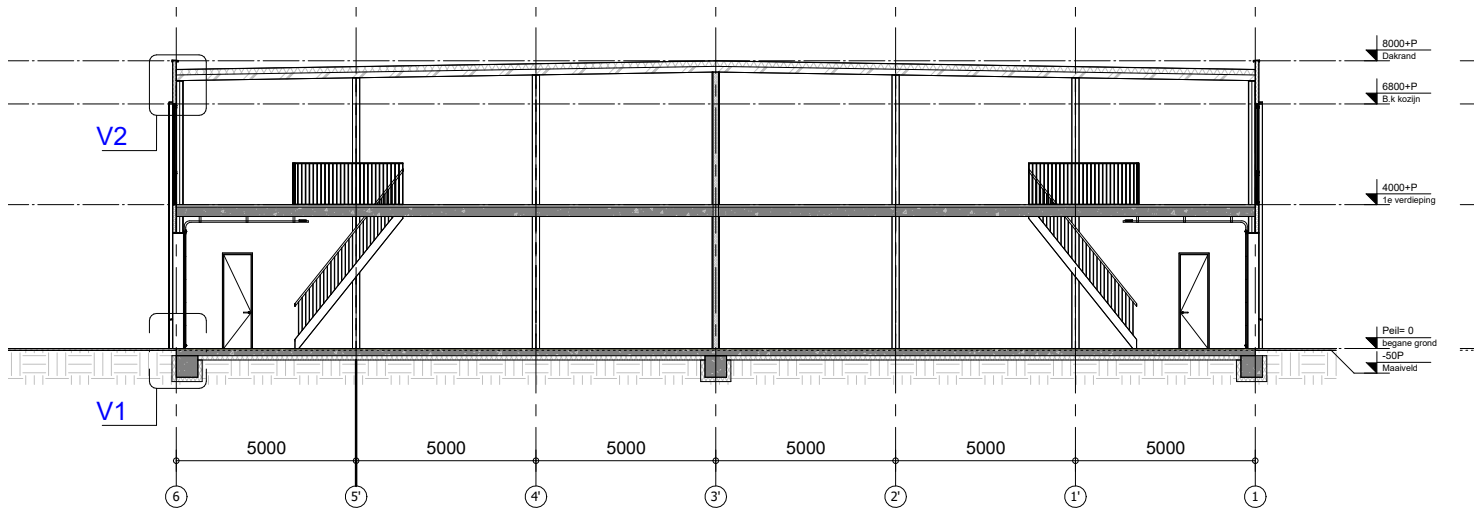
Doorsnede A-A
