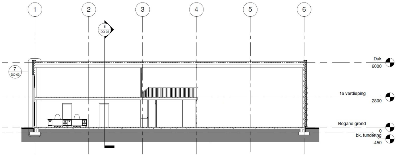
Doorsnede AA
