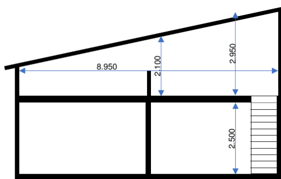
DOORSNEDE Einsteinstraat 22-24
