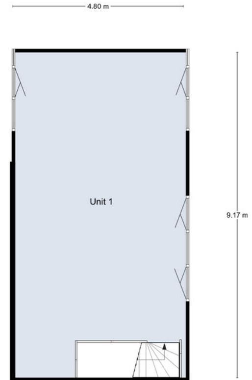
1e VERDIEPING
