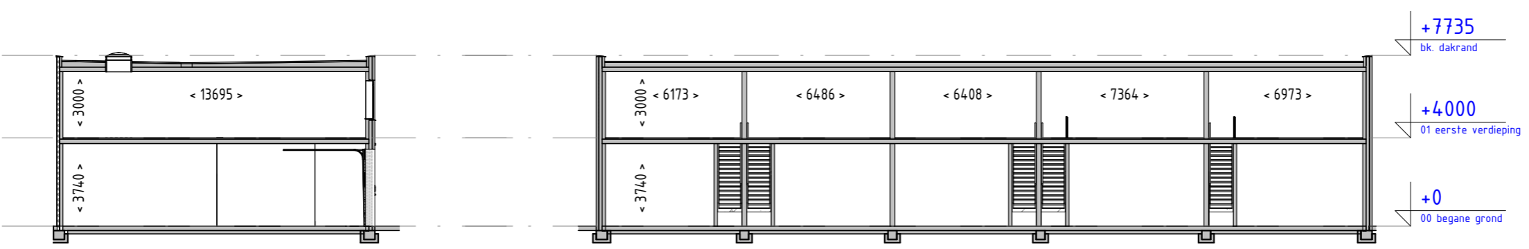
Dwarsdoorsnede
