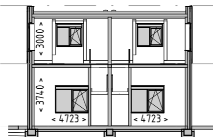
Langsdoorsnede
