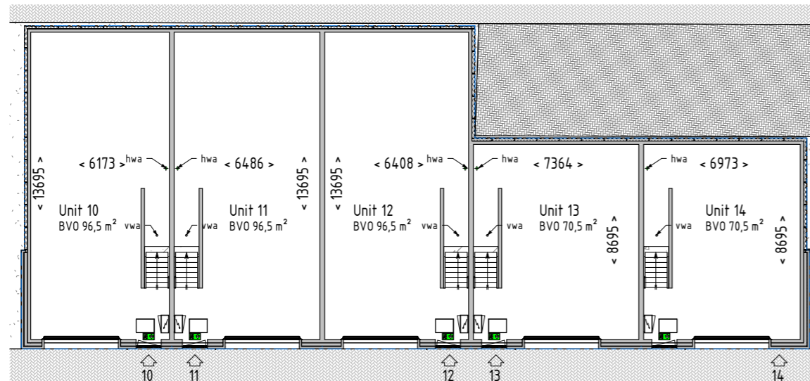
Begane grond
