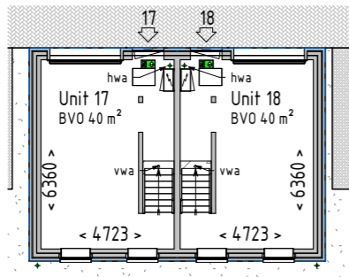
Begane grond
