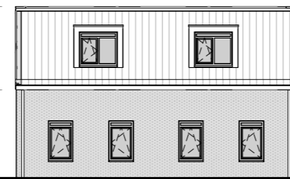
Voorgevel
