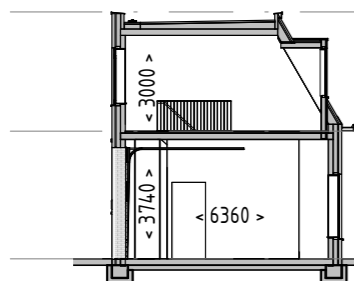
Dwarsdoorsnede
