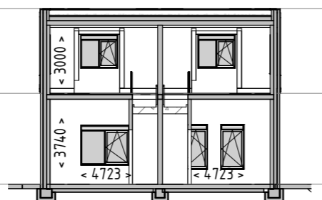
Langsdoorsnede
