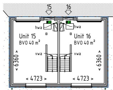
Begane grond
