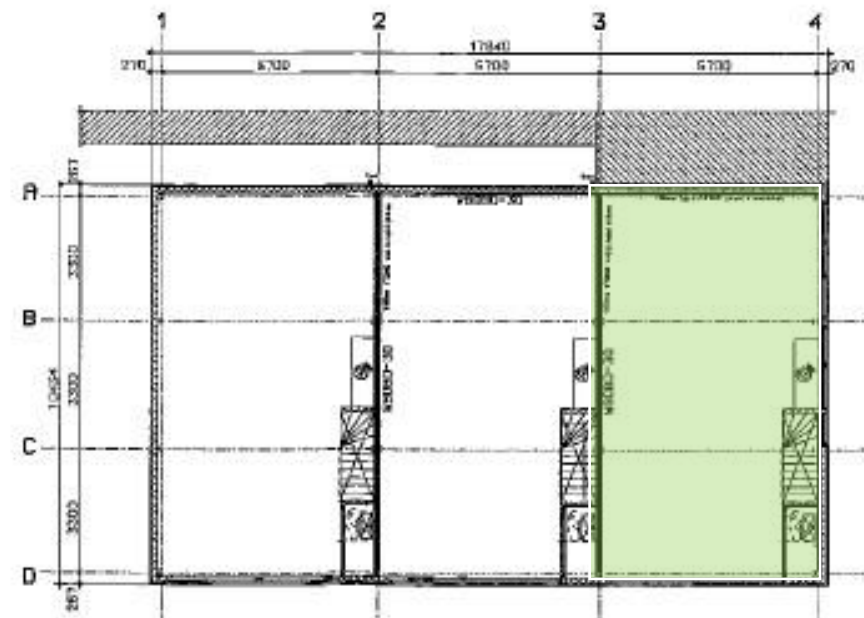
plaattegrond verdieping
