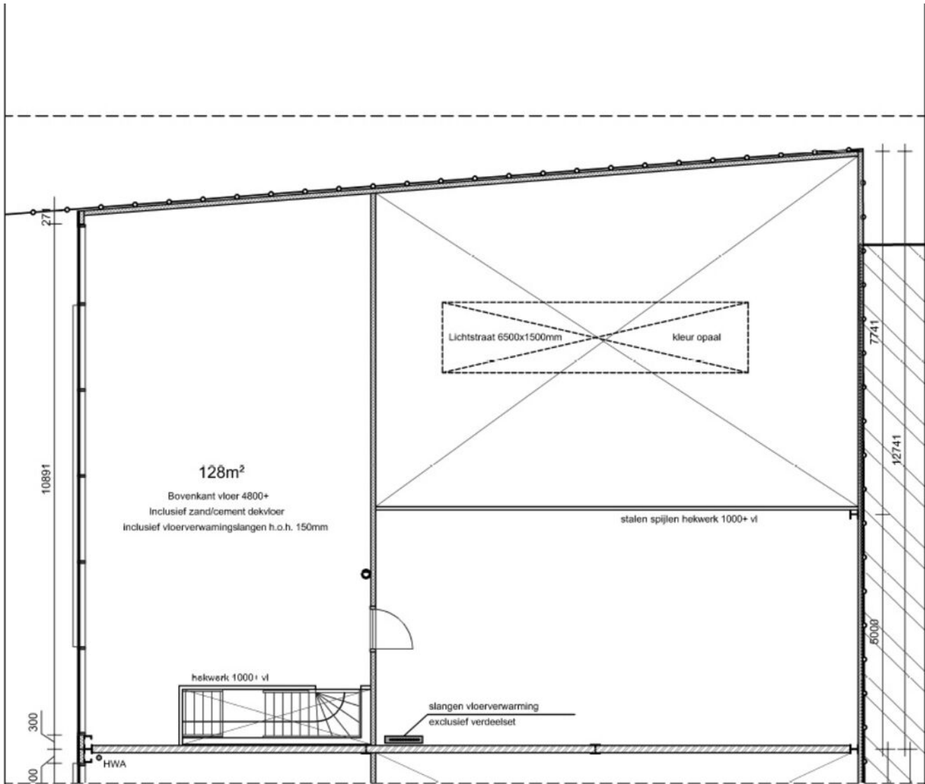
Eerste verdieping
