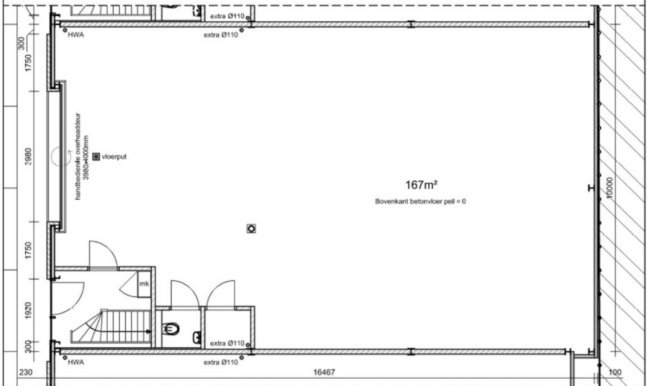
Begane grond
