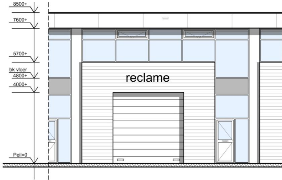
Voorgevel
