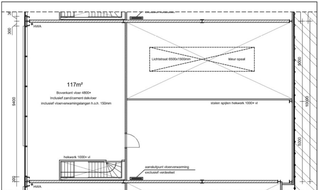
Eerste verdieping
