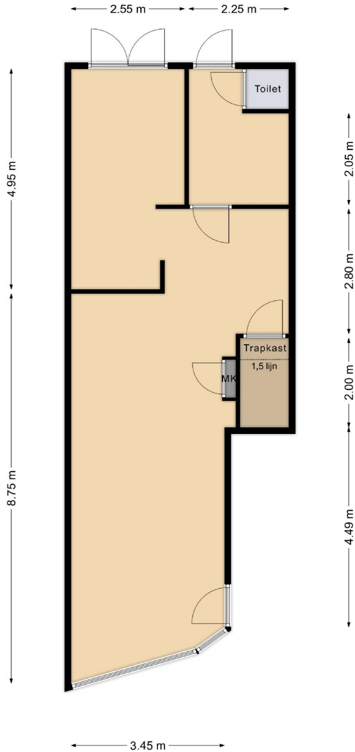
Geversstraat 59 te Oegstgeest Begane grond Indeling/maatvoering kan afwijken
