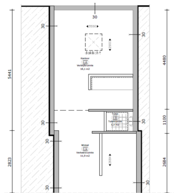
Begane grond - nieuw Vervolg
