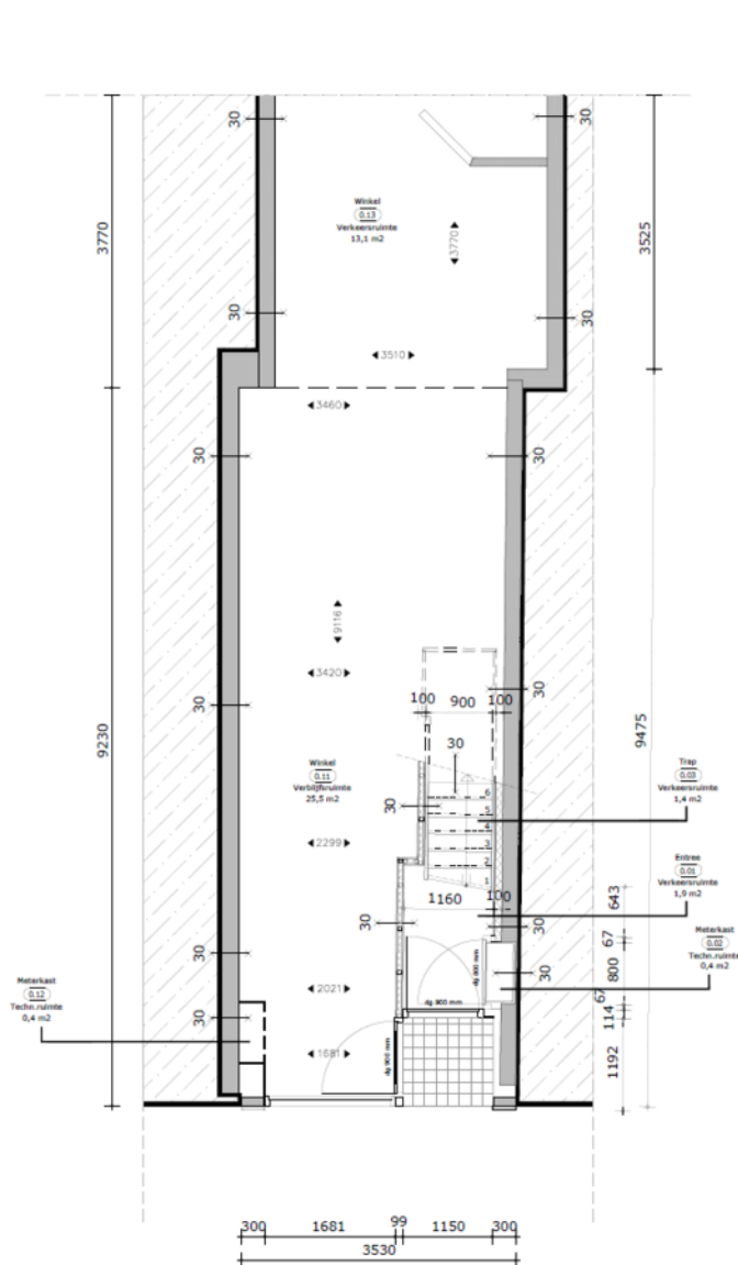
Begane grond - nieuw Peil=0
