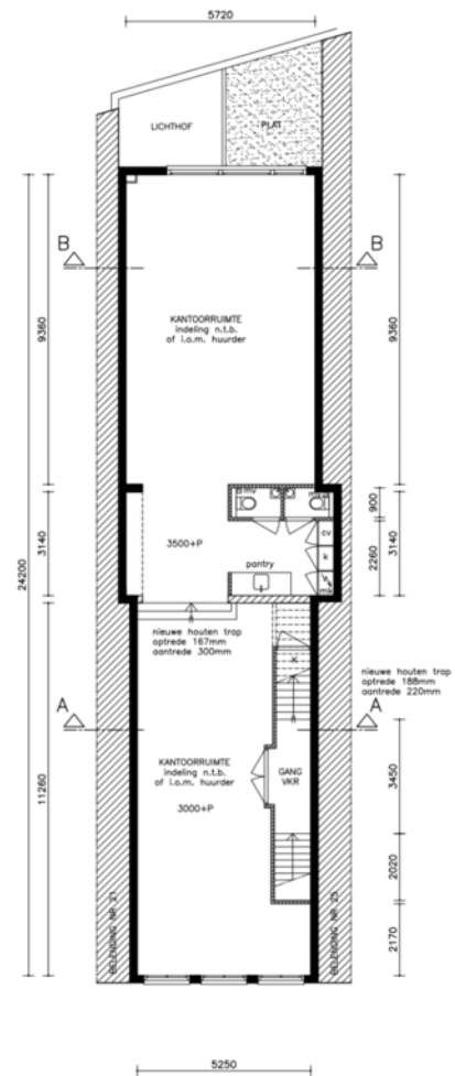
1e VERDIEPING
