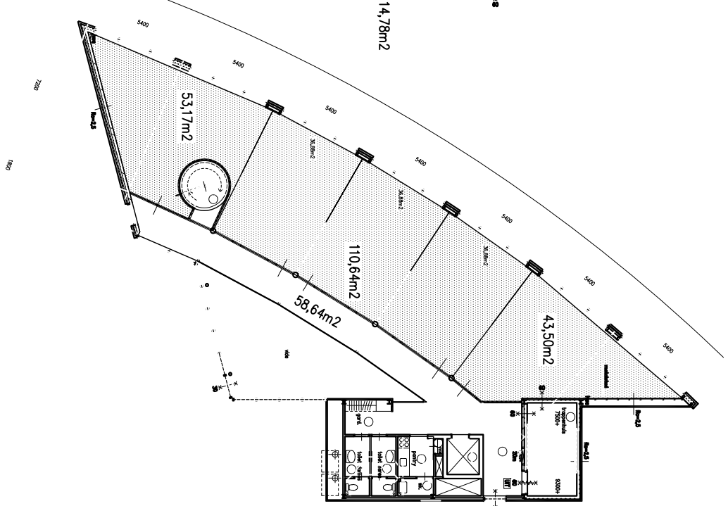
2e verdieping
