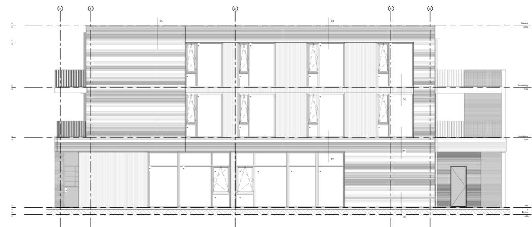
WESTGEVEL
