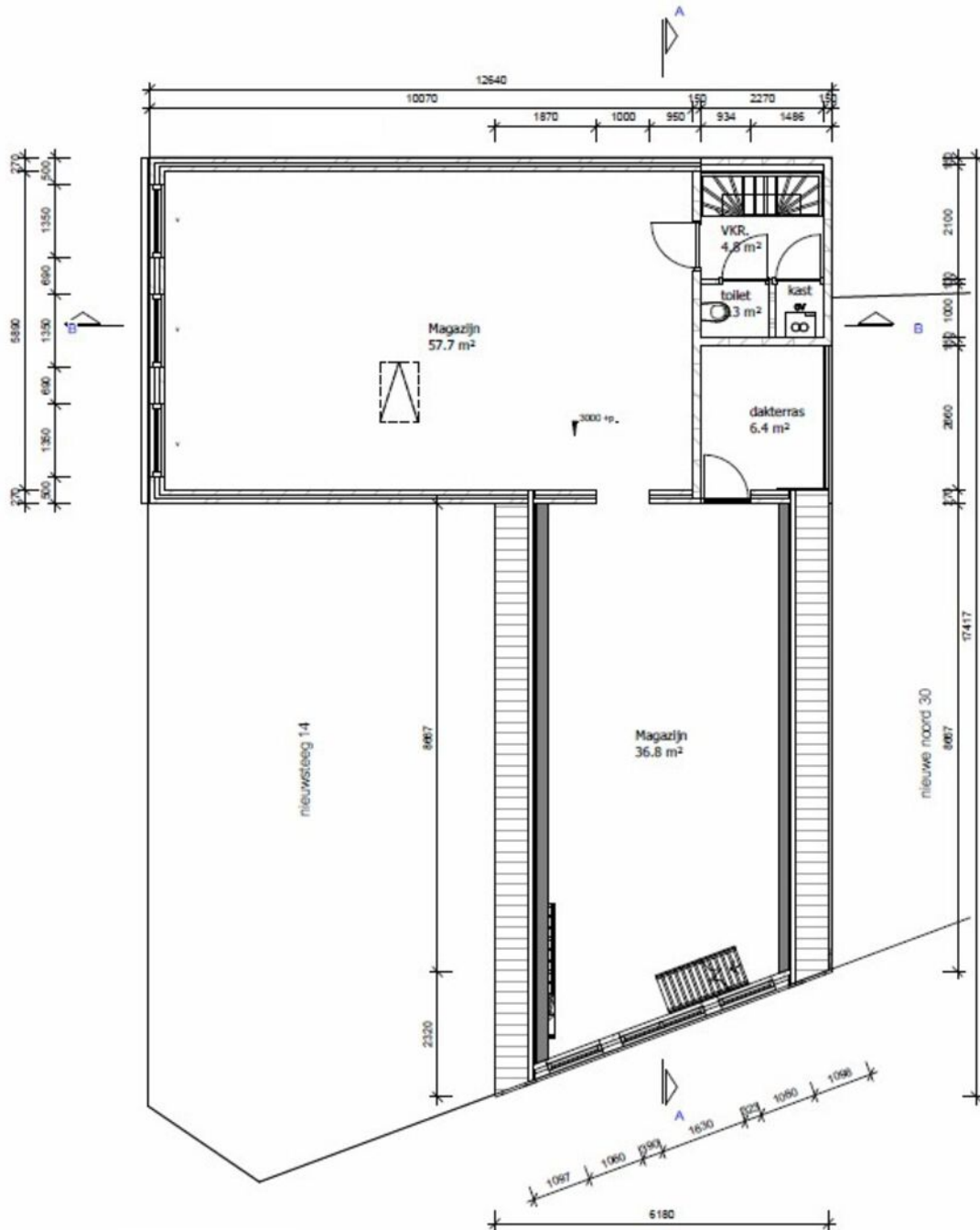
1e verdieping
