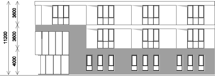
GEVEL WOUDWETERING (WESTGEVEL)
