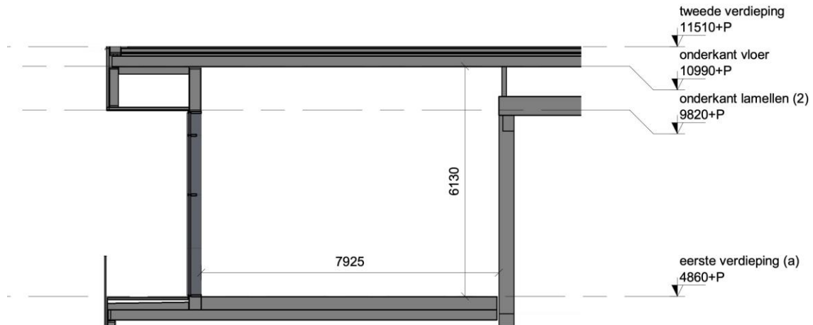
Doorsnede A-A
