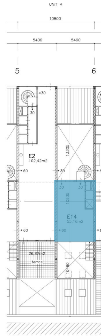
2e verdieping
