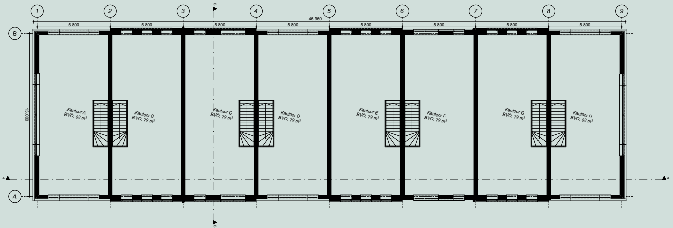
VERDIEPING
