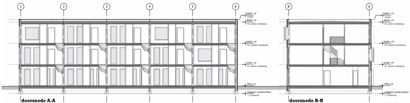
doorsnede A-A
