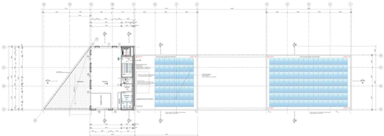
Plattegrond 2e verdieping op 7600+P
