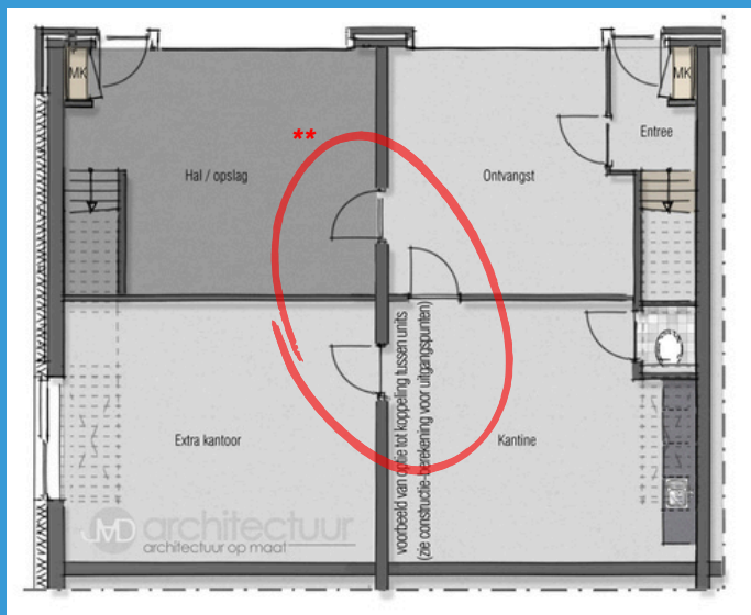
BEGANE GROND
