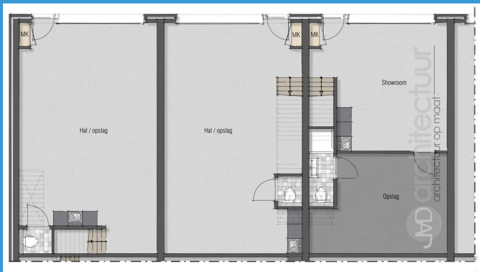
BEGANE GROND
