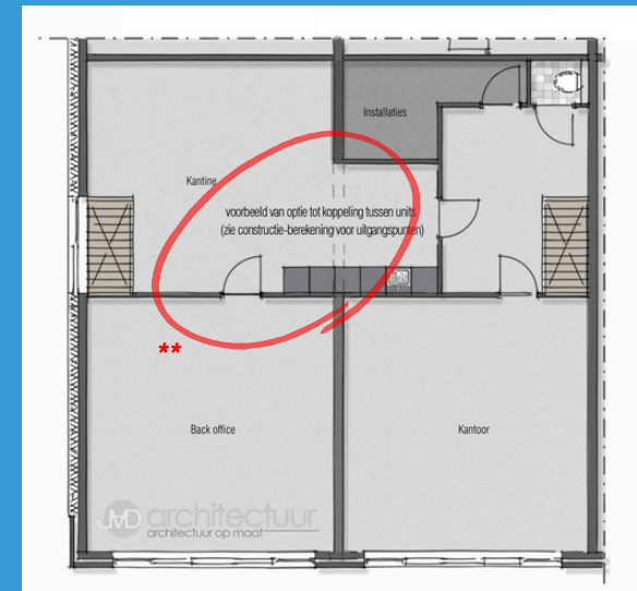
VERDIEPING
