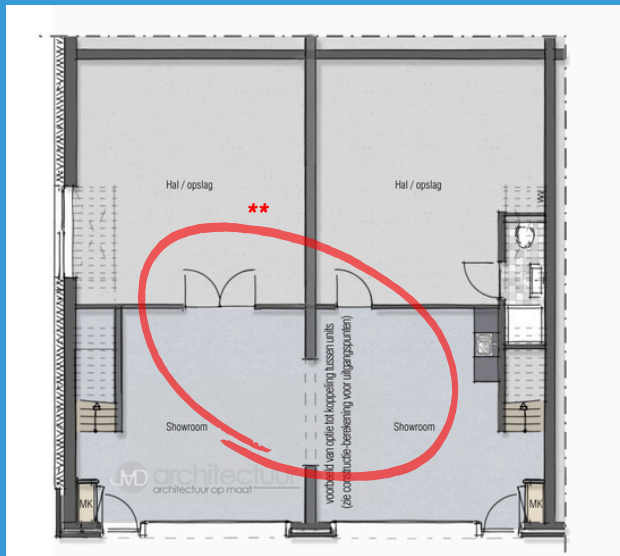
BEGANE GROND
