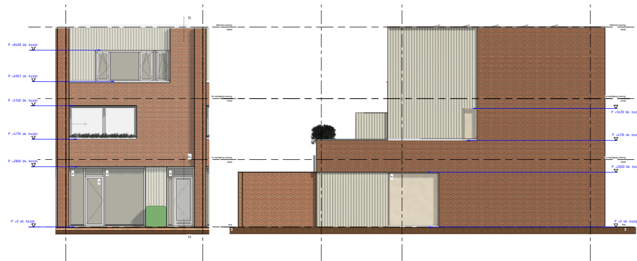
NOORDGEVEL
