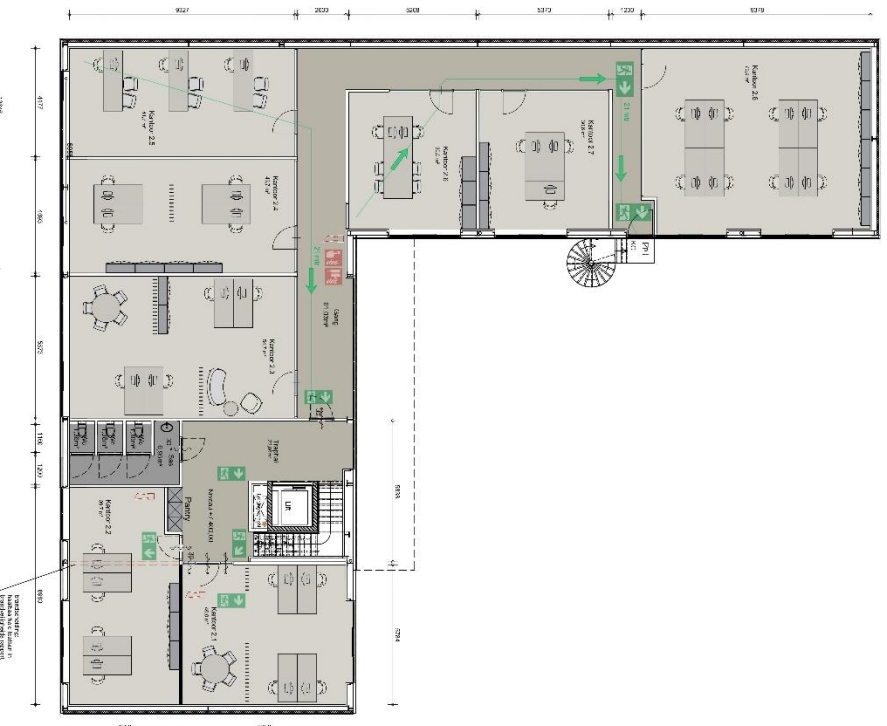
2e VERDIEPING
