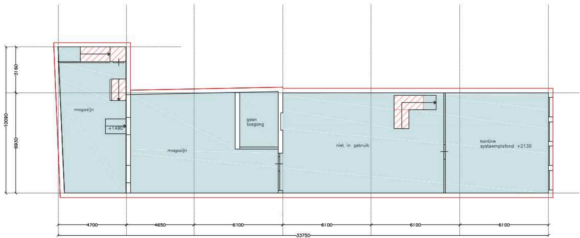
BOUWLAAG 2 – 1e VERDIEPING
