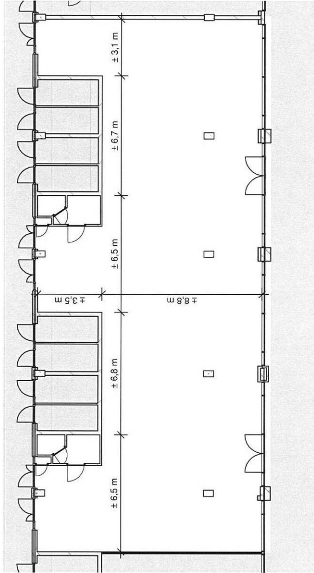
plattegrond schaal 1 : 200
