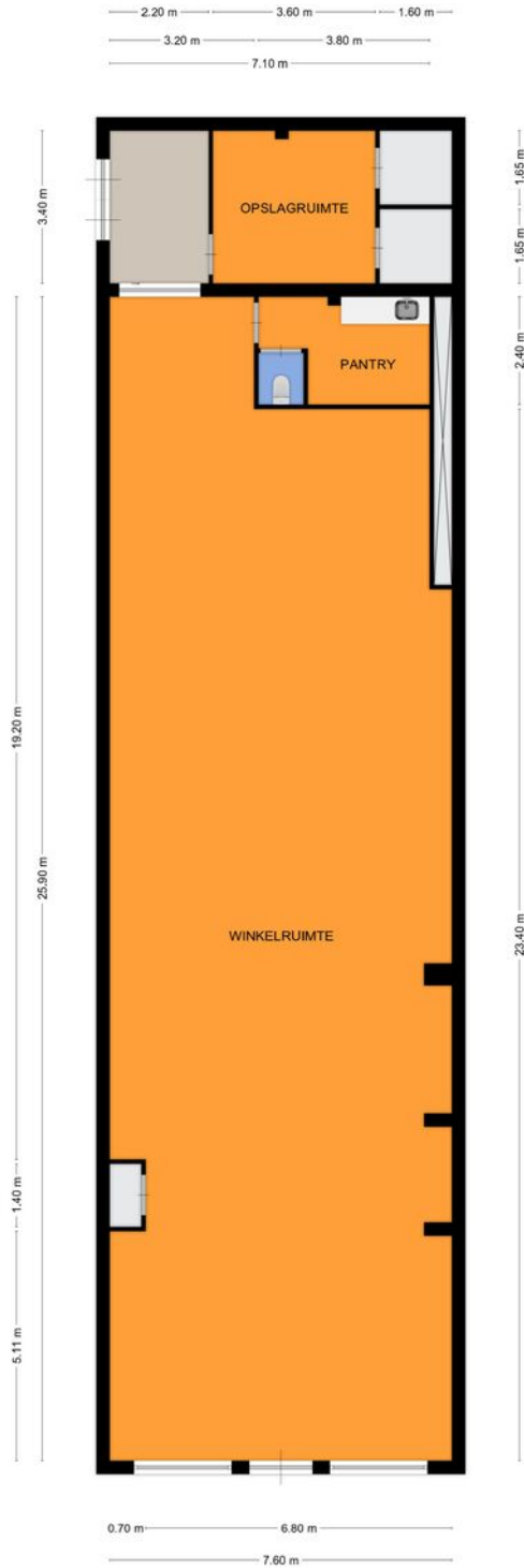
Hoogstraat 7 te Wageningen Begane Grond
